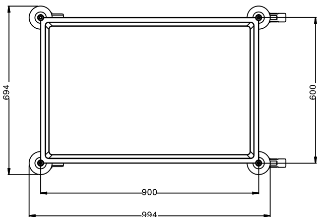
Boven aanzicht
